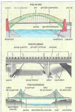
Trei tipuri clasice de planuri de poduri
