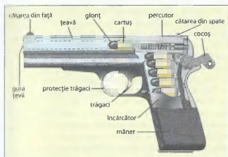
Principalele componente ale unui pistol semiautomat
