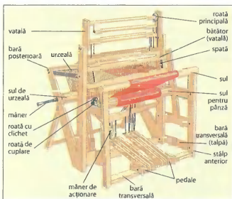
Părțile principale ale unui război de țesut manual tradițional
