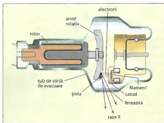
Tub cu raze X. Electronii „vaporizează” catodul când filamentul este încălzit de un curent electric. O tensiune înaltă între catod și anod determină accelerarea electronilor spre anod, care se rotește pentru a evita supraîncălzirea anticatodului. Când electronii ciocnesc anticatodul, acesta emite radiații X.
